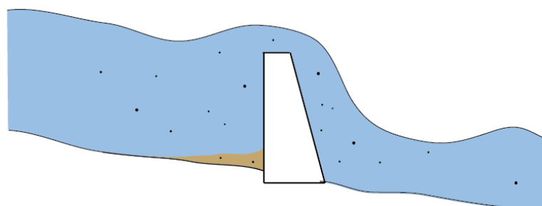
Figure 12. A) En période de basses eaux, la charge sédimentaire grossière est stockée en amont de l'ouvrage, (B) En période de hautes eaux les seuils sont dits « noyés », et sont alors partiellement ou totalement transparents au transport solide.
