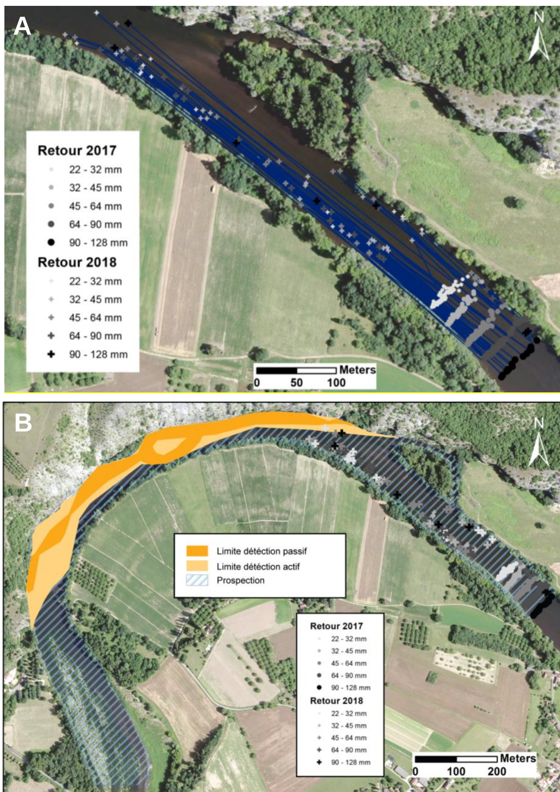
Figure 35. A - Localisation des galets équipés lors des suivis réalisés en 2017 et 2018 et déplacements des particules mises en mouvement lors de l'épisode morphogène de janvier 2018 sur le site de Meyraguet et B – Surface prospectée et zone en limite de détection pour les antennes passive et active.
