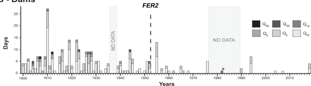
Figure 27. Chroniques des événements potentiellement morphogènes à la station hydrométriques d'Argentat (A) en régime naturel sans influence des barrages (B) en régime influencé par les barrages (Sources : DREAL & EDF ; *maximum flood event from the newspaper).
