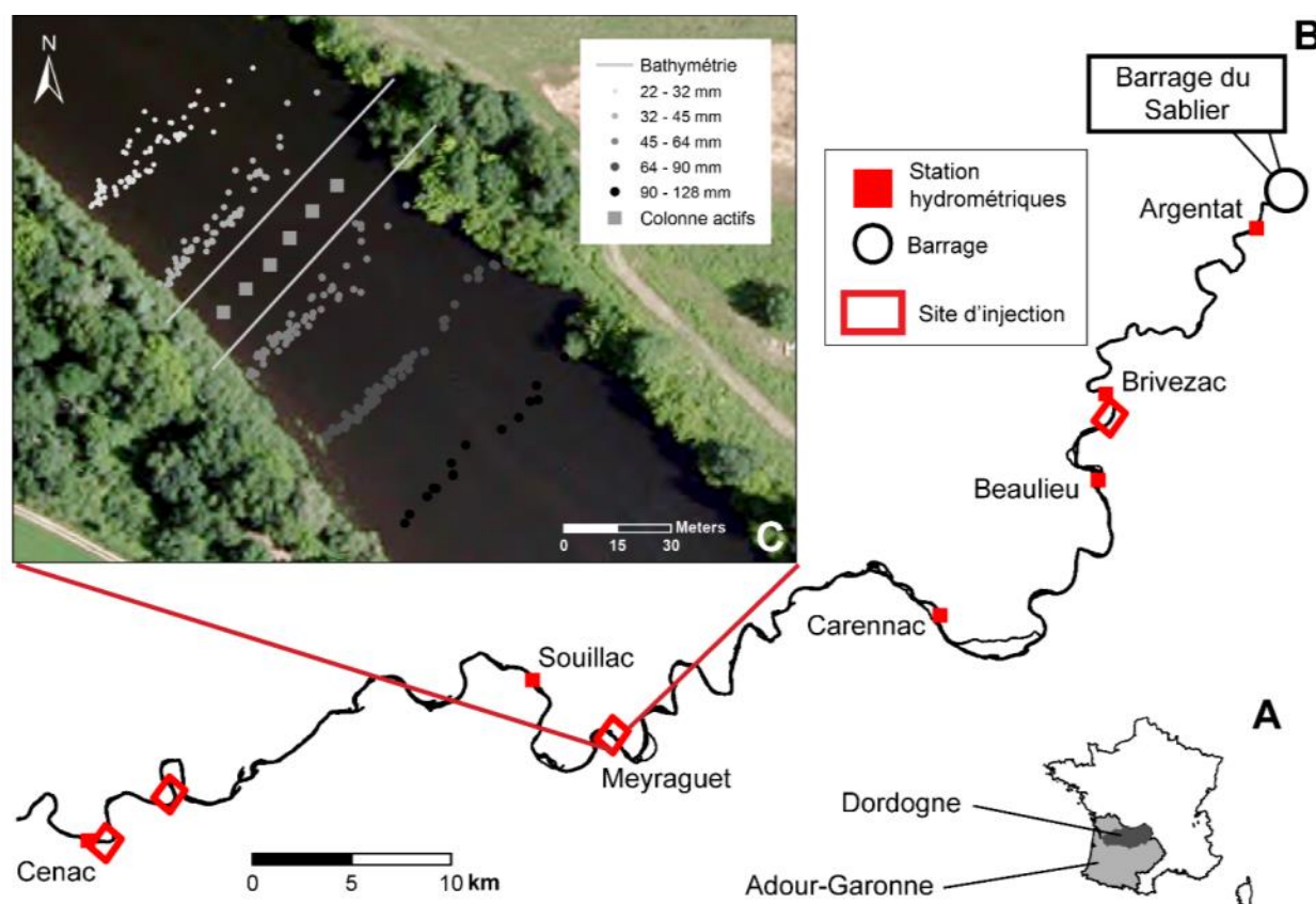
Figure 32. A – Bassin versant de la Dordogne sur le territoire français ; B - Localisation des sites d'injection sur la Dordogne moyenne : Brivezac (Corrèze – 19), Meyraguet (Lot – 46), Vitrac et Cénac (Dordogne – 24) ; C – Installation pour le suivi sédimentaire par RFID passifs et actifs sur le site de Meyraguet.
