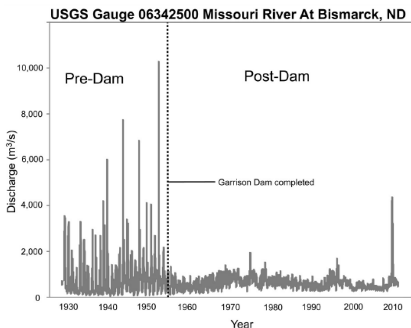
Figure 13. Débits liquides sur le Missouri (Etats-Unis) à Bismarck (aval du barrage) avant et après la construction du barrage de Garrison (d'après Shalak et al., 2013).
