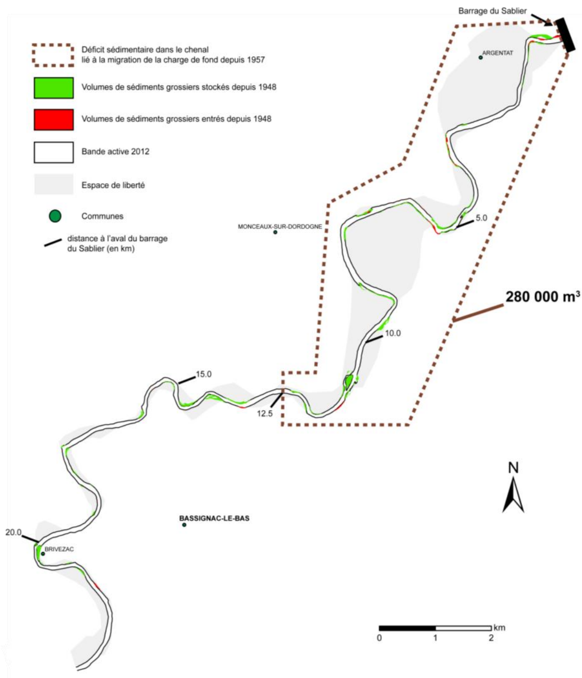
Figure 54. Cartographie de la propagation du déficit sédimentaire amont et des entrées et stockages sédimentaires depuis 1948 sur le secteur entre Argentat et Altiliac (entre 0 et 23.5 kilomètres en aval du barrage du Sablier).
